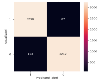
Fig. 3. Confusion Matrix.
